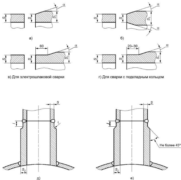
Рисунок 14 - Стыковка элементов разной толщины
