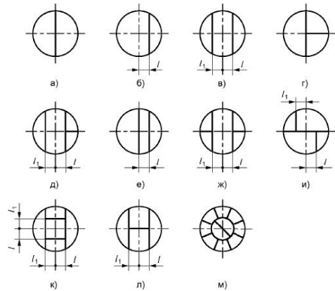
Рисунок 1 - Расположение сварных швов заготовок выпуклых днищ
