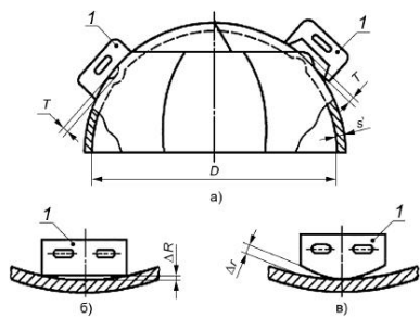
Рисунок 7 - Отклонение формы полусферического дна
