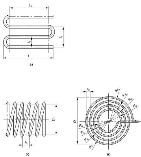
Рисунок 12 - Размеры гнутых змеевиков
