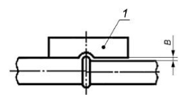
Рисунок 10 - Схема определения смещения кромок стыкуемых труб
