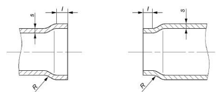
Рисунок 5 - Отбортованный и переходный элементы
