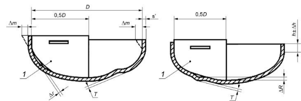
Рисунок 6 - Отклонение размеров и формы эллиптического днища
