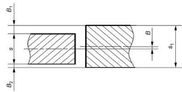
Рисунок 15 - Смещение кромок
