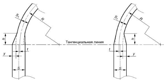
Рисунок 2 - Узел соединения днища с обечайкой
