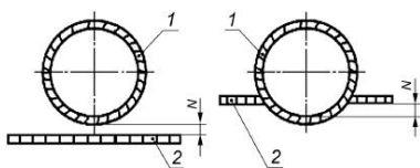
Рисунок 9 - Расстояние N
