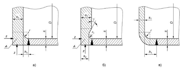
Рисунок 4 - Плоские днища
